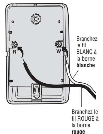
Panneau de commande MyQ®
